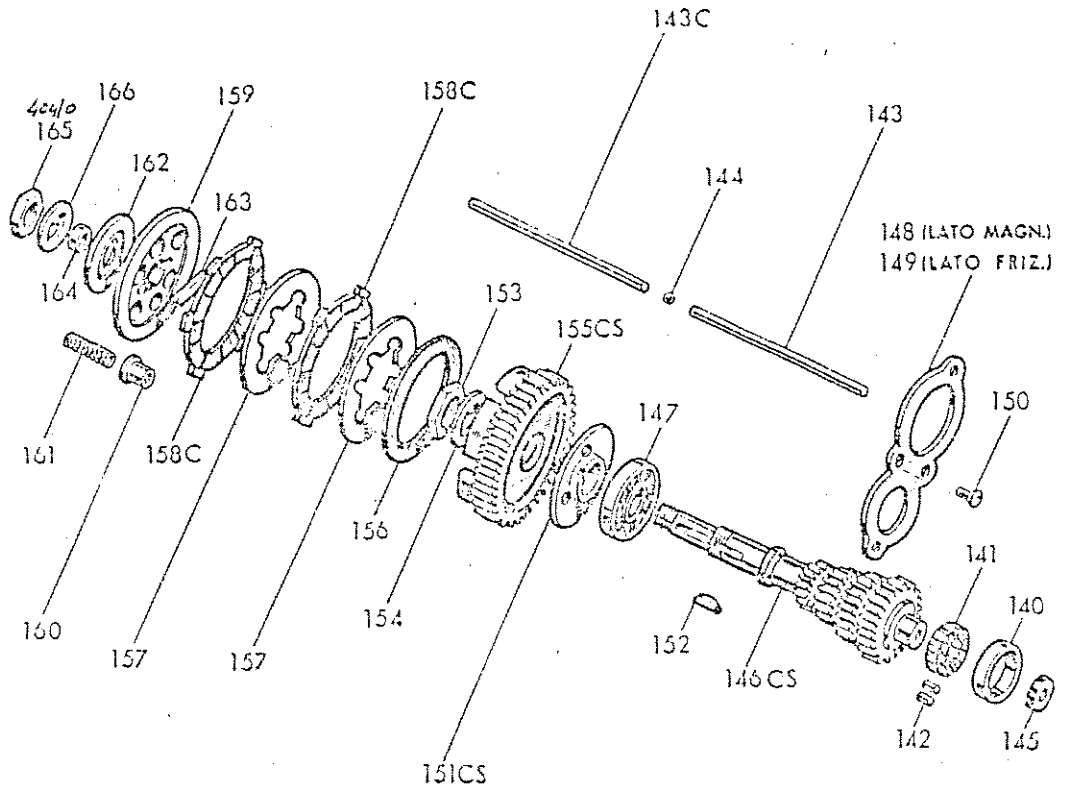
6 - ALBERO FRIZIONE - SPORT 4 MARCE
